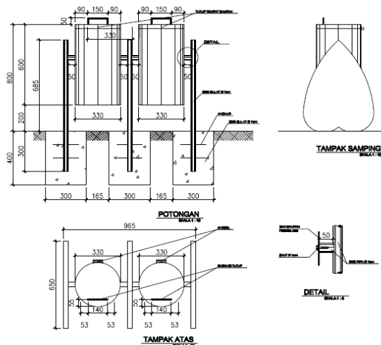
Gambar 26 Detail dan Potongan Tempat Sampah 1 (Sumber: Peneliti)
