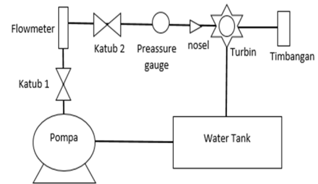
Gambar 3.2 Skema pengujian eksperimental sudu-sudu turbin
