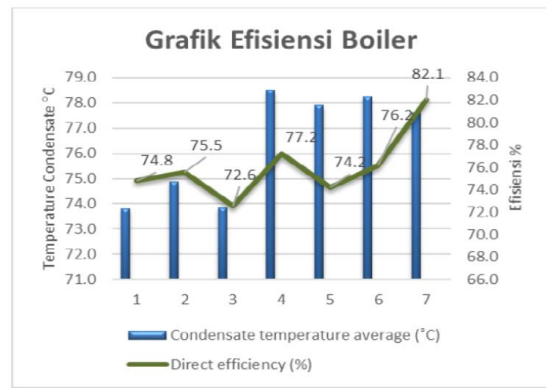
Gambar 3 Grafik efisiensi boiler setelah perbaikan
