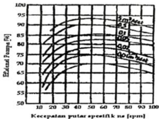
Gambar 7. Grafik efisiensi pompa
