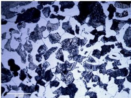
Gambar.9 Perlit (sumber: de.wikipedia.org)
