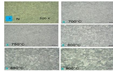
Gambar.20 Perbandingan metalografi pada titik 3 dari masing-masing sampel.
