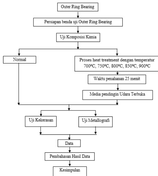
Gambar.13. Diagram Alir Penelitian pada Outer Ring Bearing .
