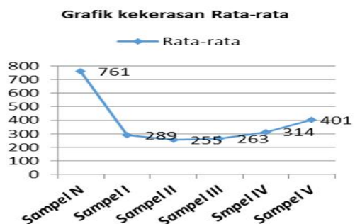
Gambar.22 Grafik rata-rata kekerasan pada titik 1, 2 dan 3 dari masing-masing sampel.
