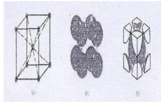
Gambar.5. Bentuk sel satuan BCC (sumber: cyberships.wordpress.com)
