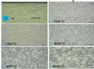
Gambar.18 Perbandingan metalografi pada titik 2 dari masing-masing sampel.
