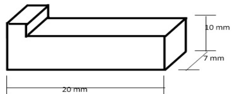
Gambar.14 Specimen Benda Uji. (Sumber: B2TKS Puspitpek-Serpong )
