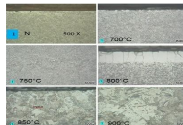
Gambar.17 Perbandingan metallografi pada titik 1 dari masing-masing sampel.
