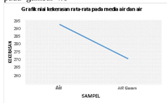
Gambar 4.6 Grafik Nilai Rata-Rata Uji Kekerasan Vickers
