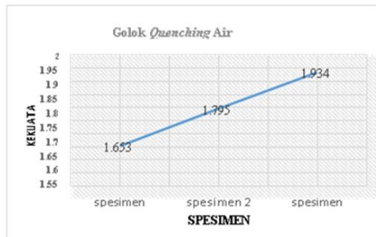
Gambar 4.7 Grafik Uji Impact Pada Golok Quenching Air
