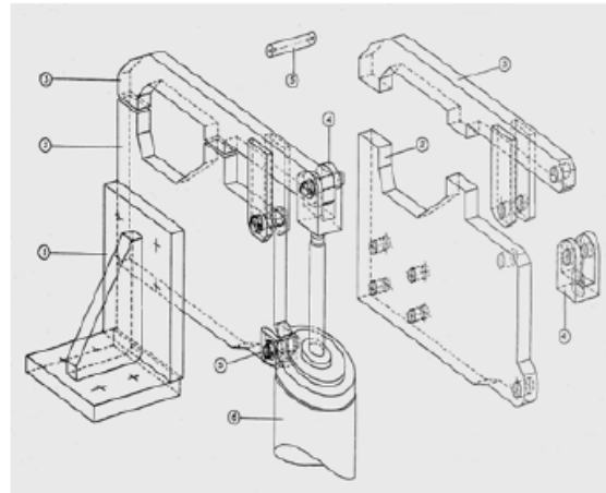
Gambar 3.3. Locator Tipe C
