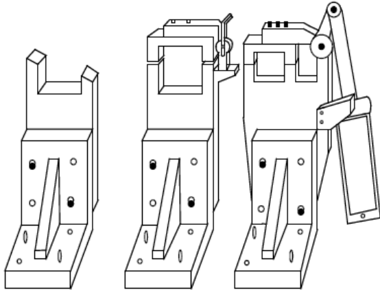
Gambar 2.5. Locator tipe A, B, C
