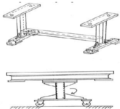
Gambar 2.3. Fixed dan rotary stand
