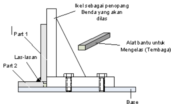
Gambar 4.1. Material yang sedang dilas
