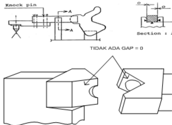
Gambar 3.14. Posisi Stopper Pin dan Arm Clamp
