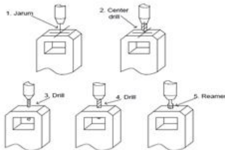
Gambar 4.2. Pembuatan lubang pin
