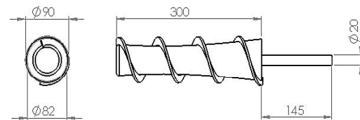
Gambar 5. Poros ulir
