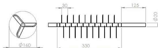
Gambar 4. Pisau Pencacah
