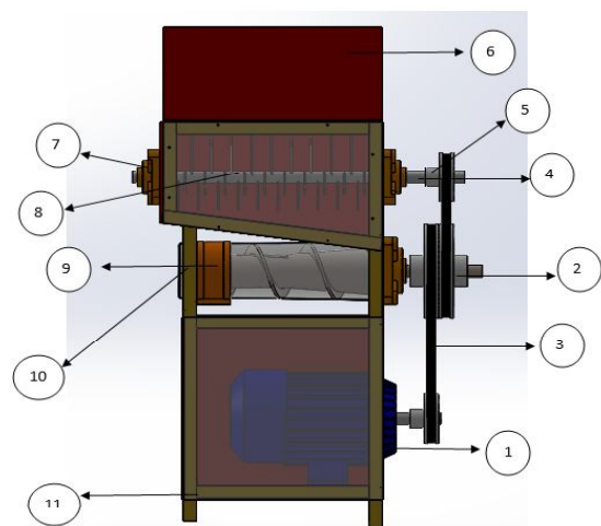
Gambar 2. Layout akhir Mesin Pengolah Limbah Styrofoam
