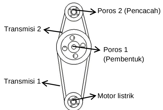
Gambar 6. Transmisi daya mesin pengolah limbah styrofoam
