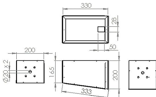
Gambar 3. Dimensi kotak pencacah
