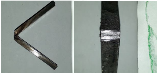
Gambar 10. Hasil benda uji impact tanpa lapisan
