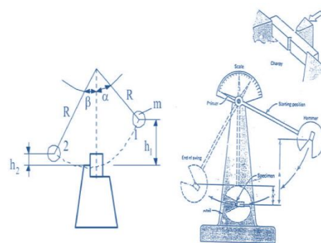
Gambar 2. Ilustrasi Skematis Pengujian Impact Charpy
