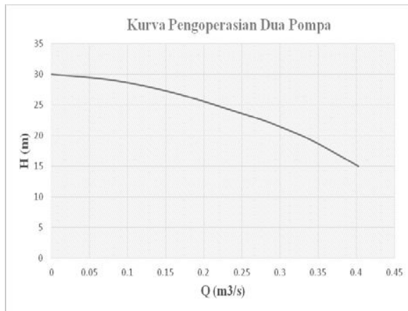
Gambar 11. Kurva karakteristik pompa gabungan
