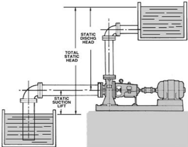
Gambar 3. Sistem kerja pompa mendatar (Sumber : http://www.agussuwasono.com/e-book/e-book-umum )
