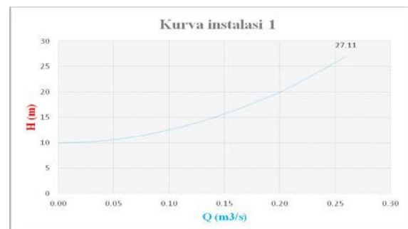
Gambar 7. Grafik sistem untuk pengoperasian satu pompa
