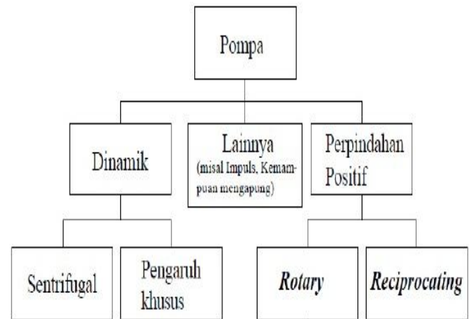
Gambar 1. Berbagai jenis pompa (Sumber: https://cimporong02.wordpress.com/dasar-dasar-pompa )
