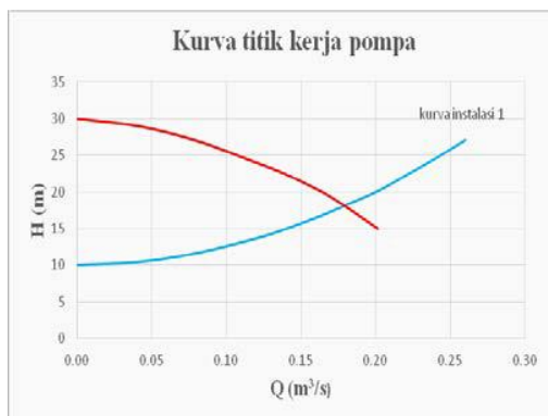
Gambar 9. Kurva titik kerja pompa dengan pengoperasian satu pompa
