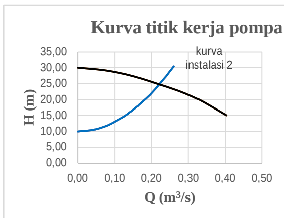
Gambar 12. Kurva titik kerja pompa dengan pengoperasian dua pompa
