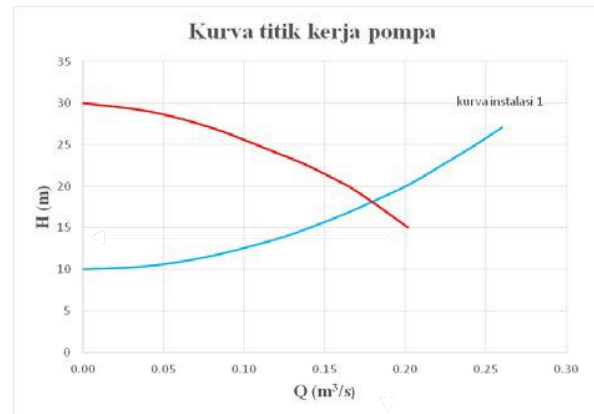
Gambar 13 Kurva titik kerja pompa dengan karakteristik instalasi 1
