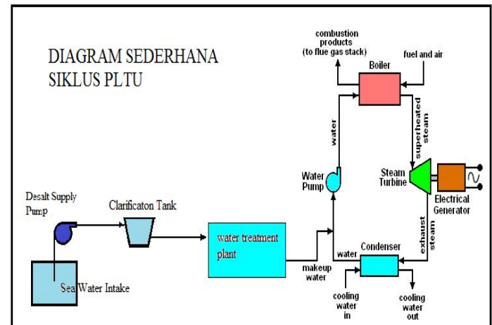
Gambar 2. Siklus fluida kerja sederhana pada PLTU
