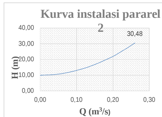
Gambar 10. Grafik sistem untuk pengoperasian dua pompa
