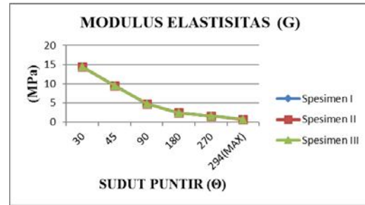
Gambar 4 Grafik Perbandingan modulus elastisitas dengan sudut puntir material aluminium 2319
