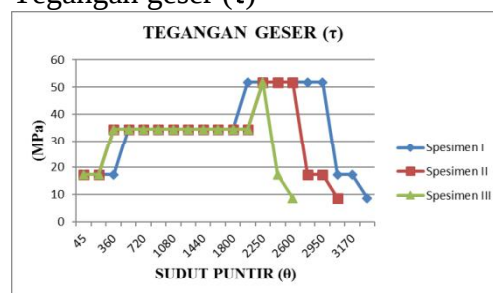
Gambar 1 Grafik Perbandingan tegangan geser dengan sudut puntir baja SS41
