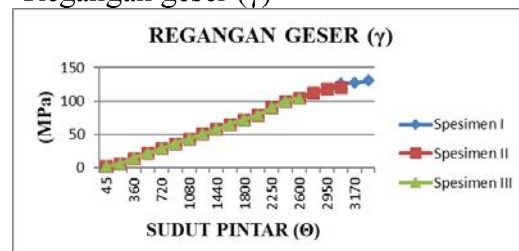
Gambar 4.5: Grafik Perbandingan regangan geser dengan sudut puntir material SS41
