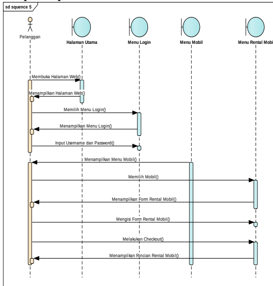
Gambar 6 Sequence Diagram Pemesanan Rental Mobil
