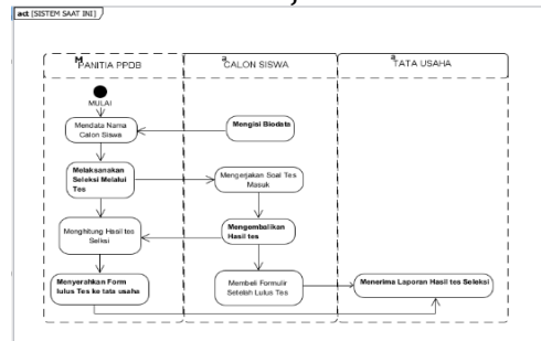
Gambar 1. Diagram Aktivitas Sistem Yang Sedang Berjalan
