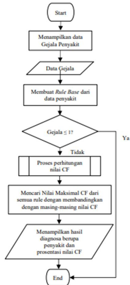
Gambar 5. Flowchart system menggunakan metode Certainty Factor
