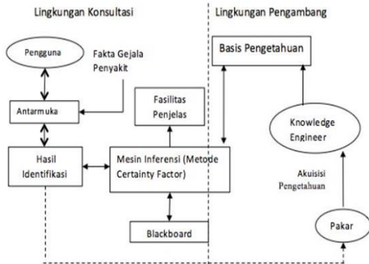
Gambar 3. Arsitektur Sistem Pakar Diagnosa Penyakit Pencernaan
