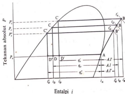
Gambar 3. Perubahan temperature pengembunan
