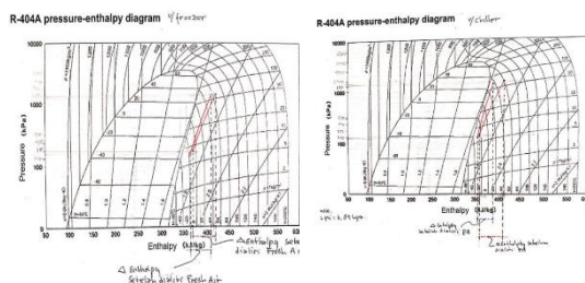
Gambar 6. Entalphy sebelum dan sesudah dialiri Fresh Air
