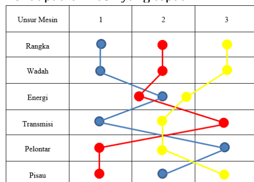
Gambar 11. Struktur Modul
