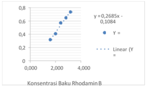
Gambar 2. Kurva Kalibrasi Larutan Rhodamin B Terhadap Konsentrasi
