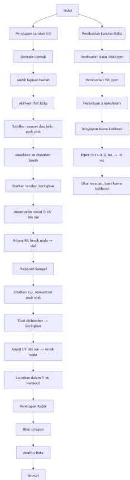
Gambar 1. Skema Penelitian
