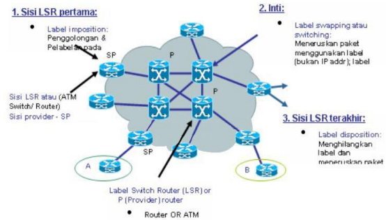
Gambar 2. Arsitektur Jaringan MPLS
