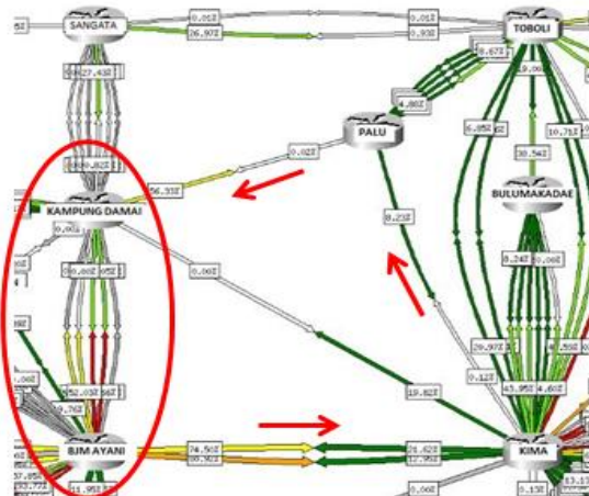
Gambar 13. Re-route LSP melalui jalur Palu <> Kampung Damai via Kimba
