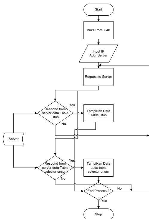
Gambar 3.3: Flowchart program pada client
