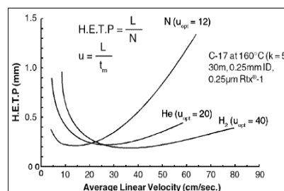
Gambar 2.2: Kurva Van Demeter untuk Hidrogen, Helium dan Nitrogen
