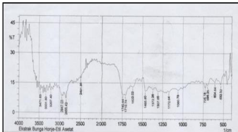
Gambar 6. Spektrum FTIR Ekstrak Etil Asetat Bunga Honje
