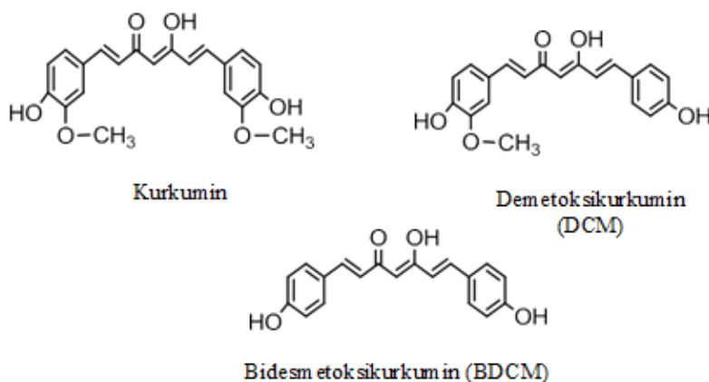
Gambar 1. Kurkumin, Demetoksikurkumin (DMC) dan Bisdemetoksikurkumin (BDMC)
