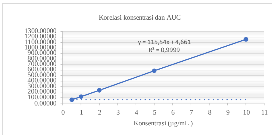
Gambar 4. Hasil uji lineritas dengan larutan seri standar
