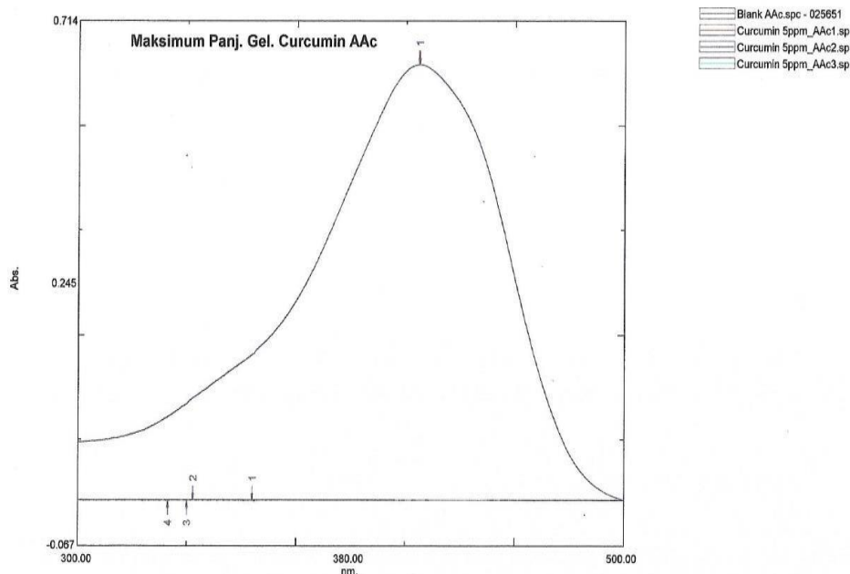
Gambar 3. Hasil pengukuran panjang gelombang kurkumin 5 µg/mL
