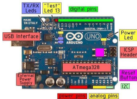
Gambar 2.1 Modul Arduino Uno
