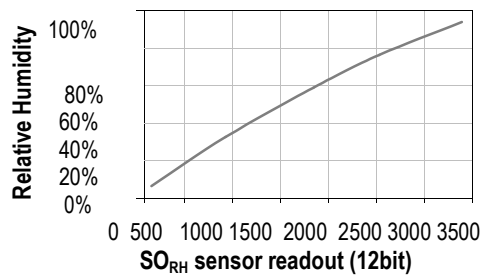
Gambar 2.2 Grafik Konversi dari SO_{RH} kelembaban relative
