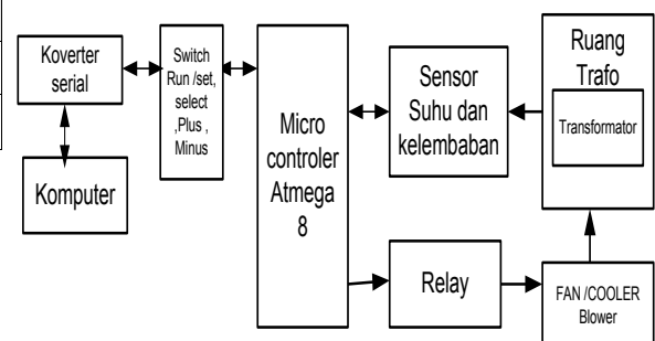
Gambar 3.1 Diagram Sistem Alur Kerja
