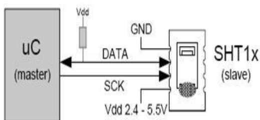
Gambar.2.1 Skema pengambilan data SHT11
