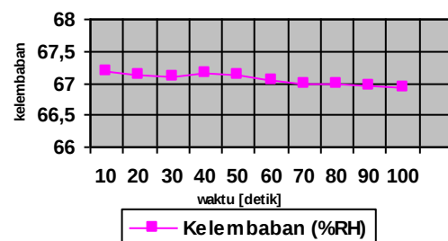
Gambar 4.5. Grafik Pengujian kelembaban tanpa beban
