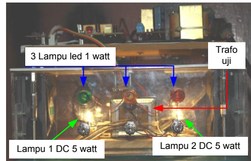
Gambar 4.1 Beban Lampu Pengujian
