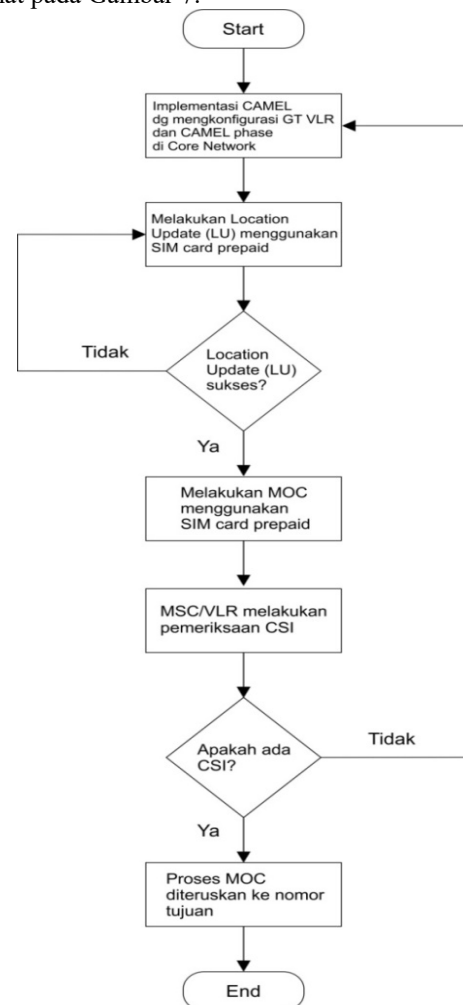
Gambar 7. Diagram alir implementasi
