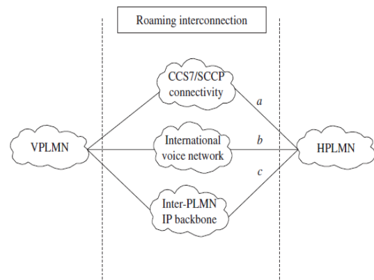
Gambar 3. Koneksi Inter-PLMN
