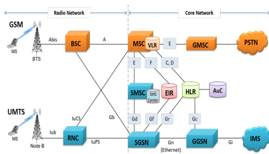
Gambar 1. Arsitektur Jaringan Seluler GSM/UMTS
