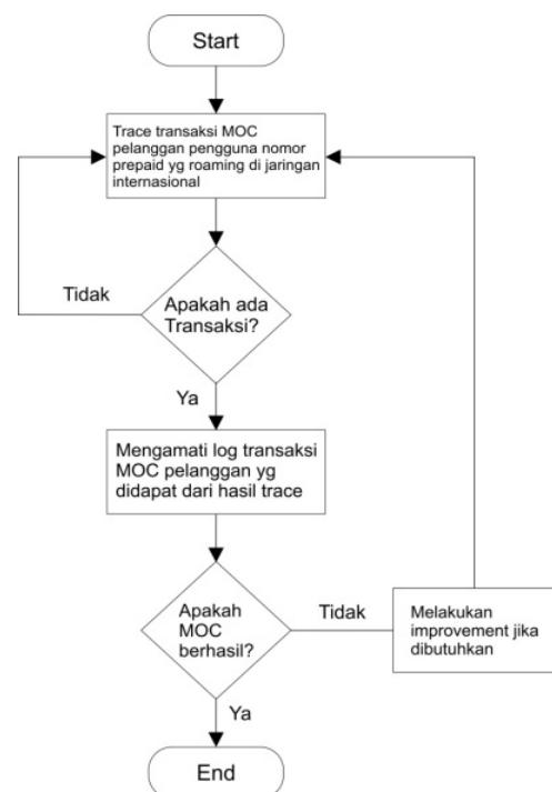
Gambar 18. Diagram Alir Pengambilan Data Transaksi MOC
