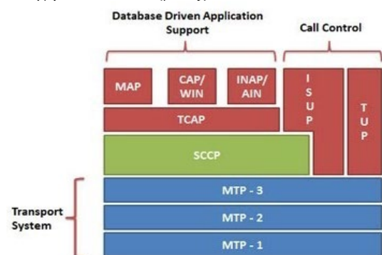
Gambar 2. SS7 layer Protocol Stack
